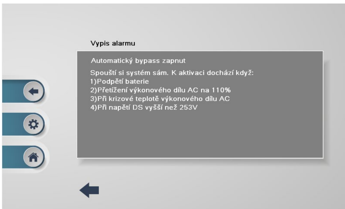
Okno Info alarmu.
