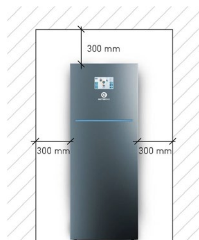
Nákres minimálních prostorových nároků pro instalaci systému CES BATTERY BOX.
