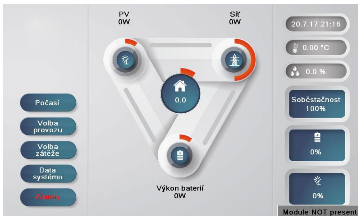
Základní obrazovka na LCD displeji systému CES BATTERY BOX.
