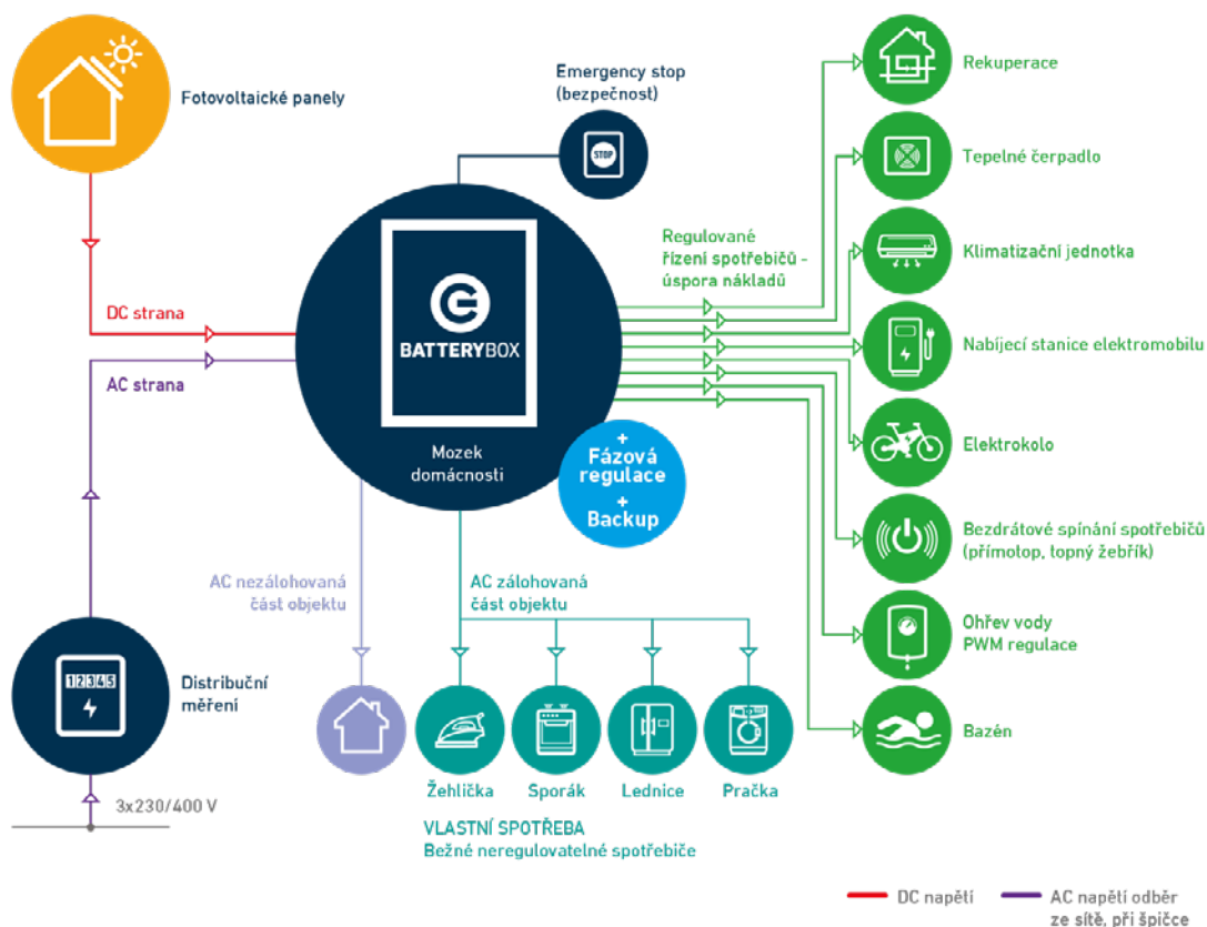
Základní schéma propojení systému CES BATTERY BOX v rámci domácnosti (AC strana, DC strana).
