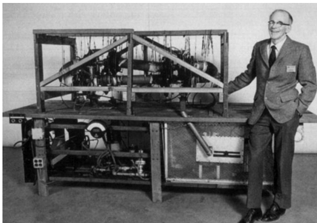
L. Spitzer pózuje před svou variantou magnetického udržení – stelarátorem. Úspěšnější byli Rusové vedením A. D. Sacharova s tokamakem.
