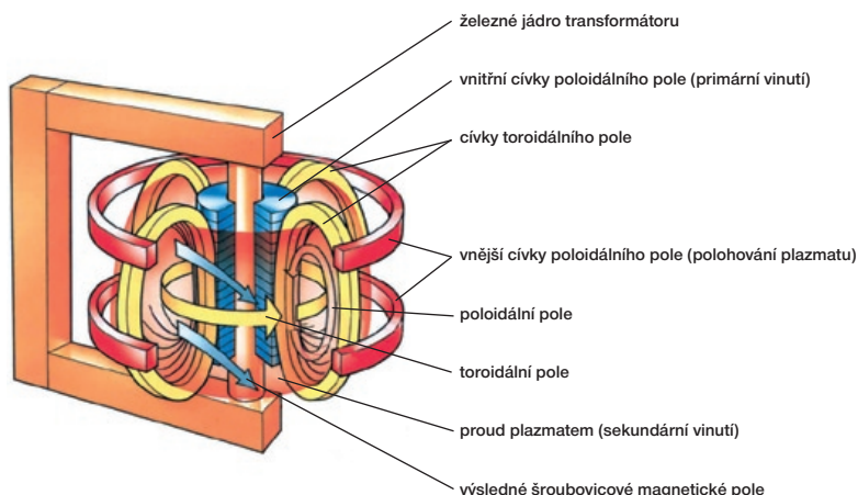
Schéma tokamaku
