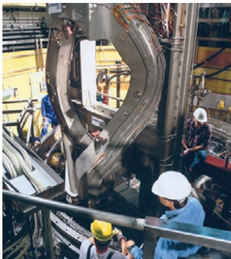
Test třídímního prototypu supravodivé cívky pro stelarátor W7-X ve Forschungszentrum Karlsruhe. Na obrázku je cívka před zapojením vsunována do kryostatů, který ji ochladí na -269\text{ }^{\circ}\text{C} .
