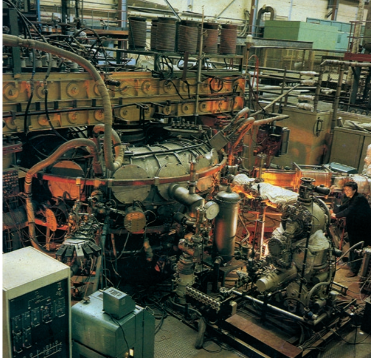
Na prvním supravodivém tokamaku na světě – moskevském T-7 – generovala v roce 1982 vlnovodná aparatura vyrobená v Ústavu fyziky plazmatu ČSAV proud 200 kA. Tehdy to byl světový rekord.
