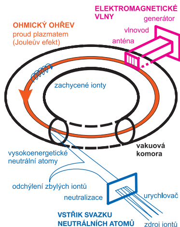
Tři metody vnějšího ohřevu plazmatu v tokamaku: základní ohmický a dodatečný s vysokofrekvenčním elektromagnetickým polem, respektive se vstřikem svazku vysokoenergetických neutrálních atomů
