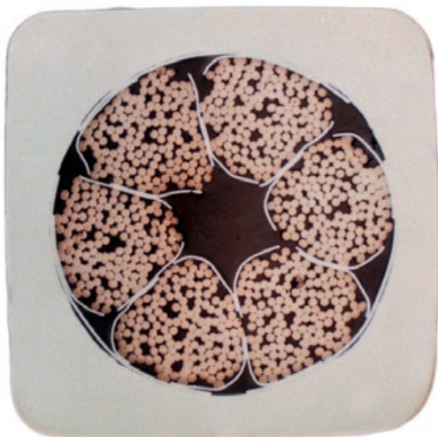
Průřez supravodičem
