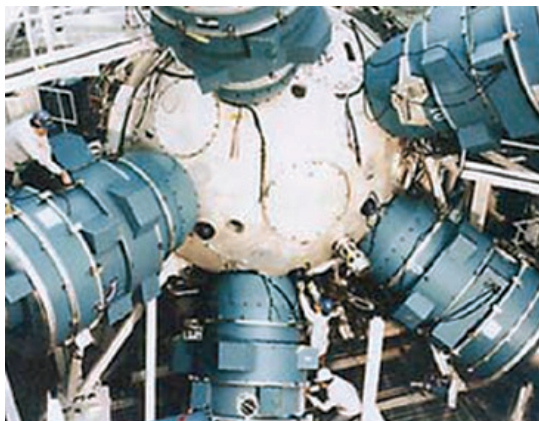
NOVA byl nejmohutnější laserový systém na světě – Lawrence Livermore National Laboratory, USA
