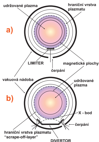
Průřez komorou tokamaku a) s limiterem, b) s divertorem. Dva způsoby jak z plazmatu odvést nečistoty, zplodiny termojaderné reakce a nespálené palivo.
