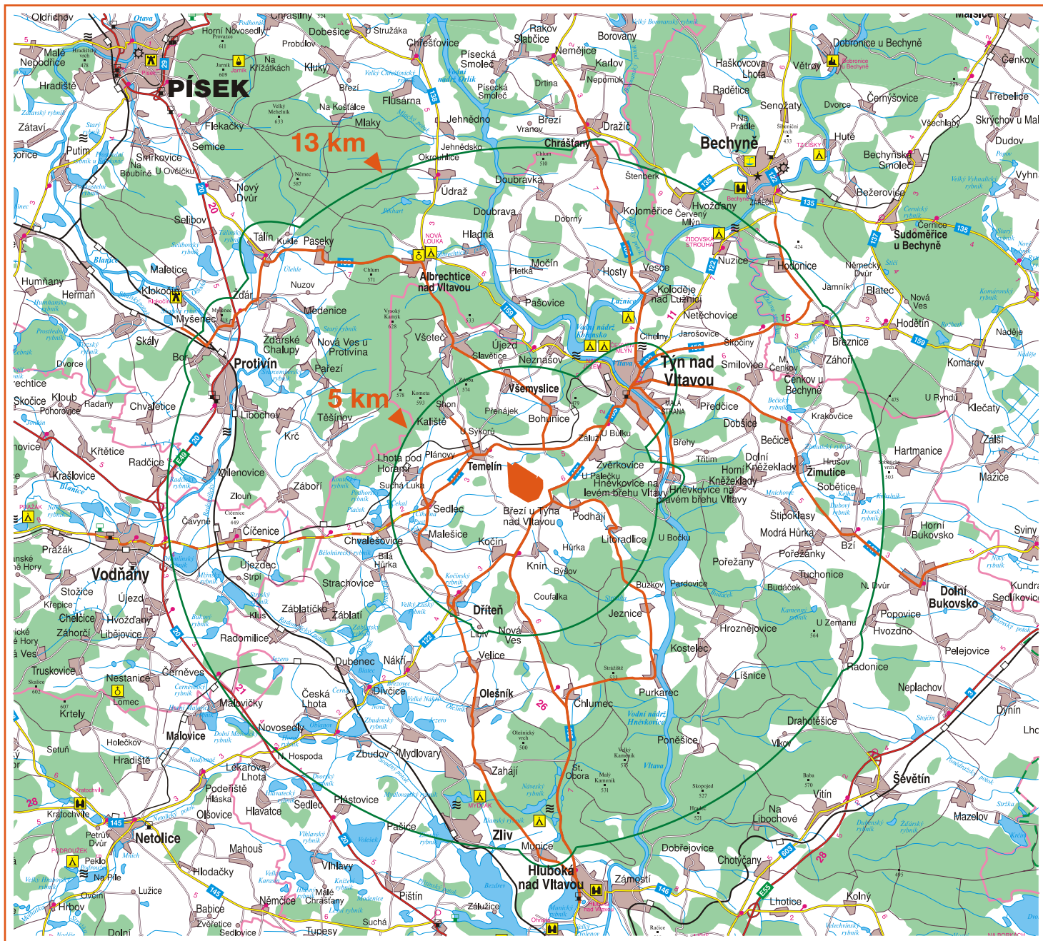
Schématické znázornění zóny havarijního plánování JE Temelín
