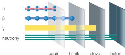
Průnik záření různými druhy materiálů
