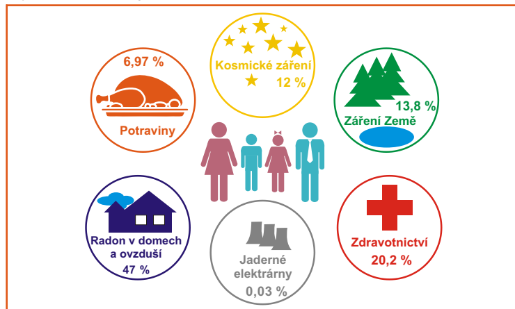
Příspěvky různých zdrojů na ozáření člověka
