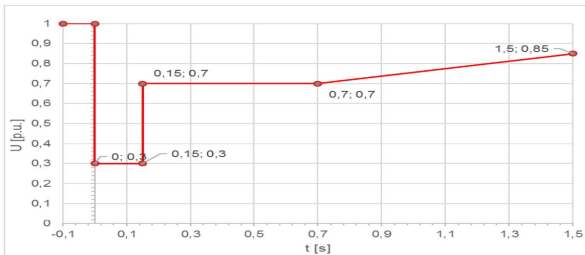
Obrázek č.4 Autonomní charakteristika FRT pro synchronní VM A1, A2, B1
