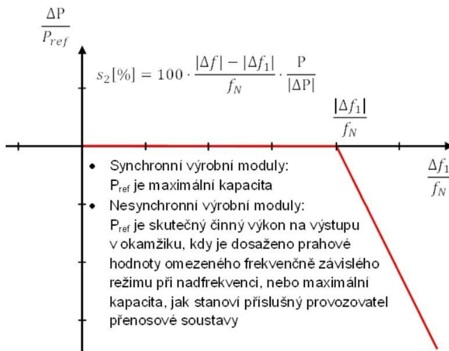
Obrázek č.2 Autonomní charakteristika P(f)
