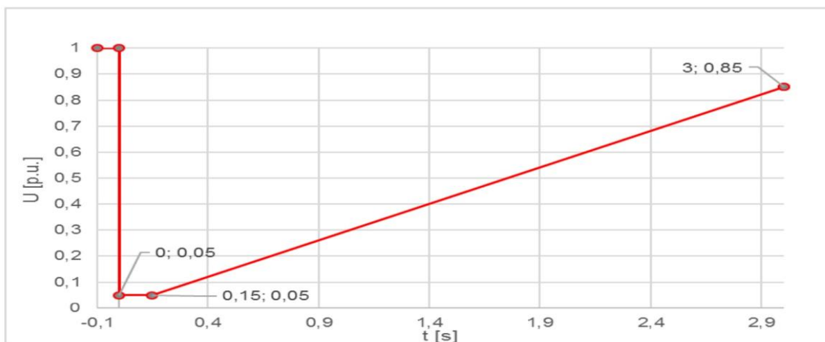
Obrázek č.3 Autonomní charakteristika FRT pro nesynchronní VM A1, A2, B2, C
