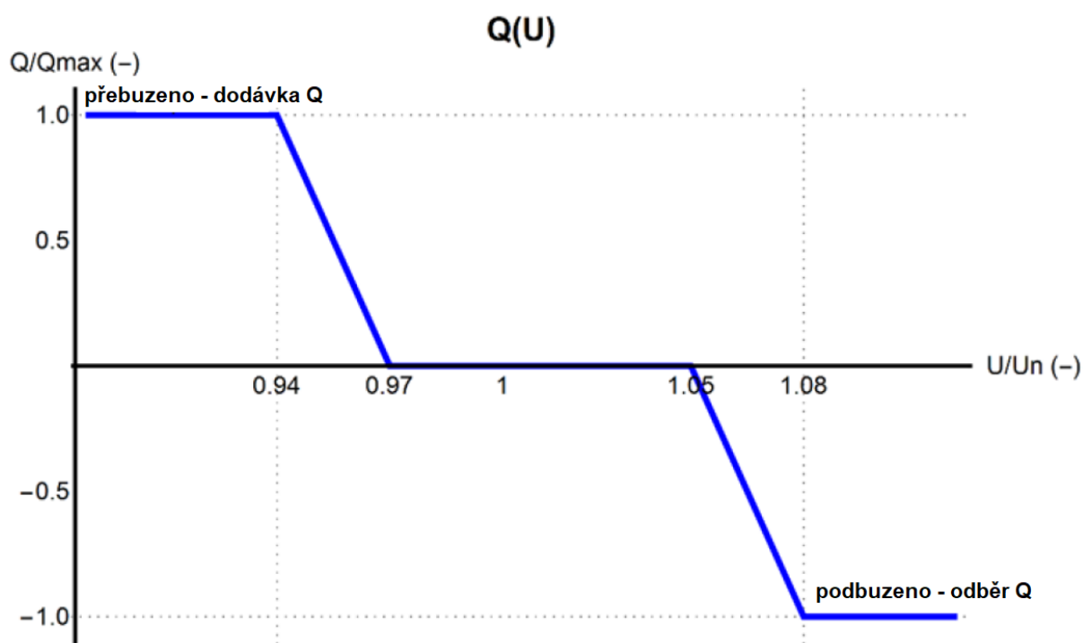
Obrázek č.1 Autonomní charakteristika Q(U)
