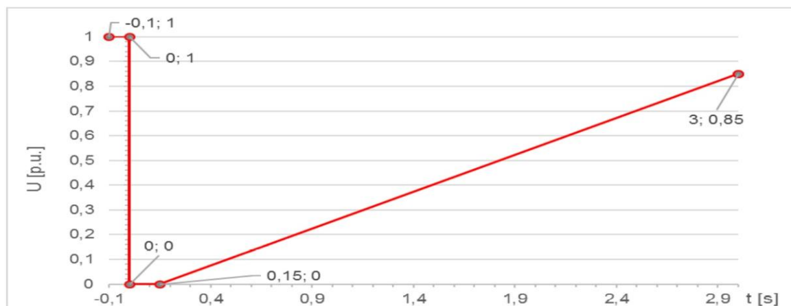
Obrázek č.7 Autonomní charakteristika FRT pro nesynchronní VM D
