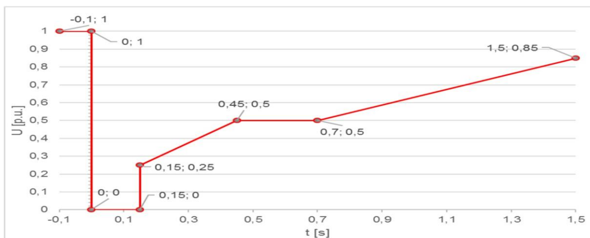
Obrázek č.6 charakteristika FRT pro synchronní VM D
