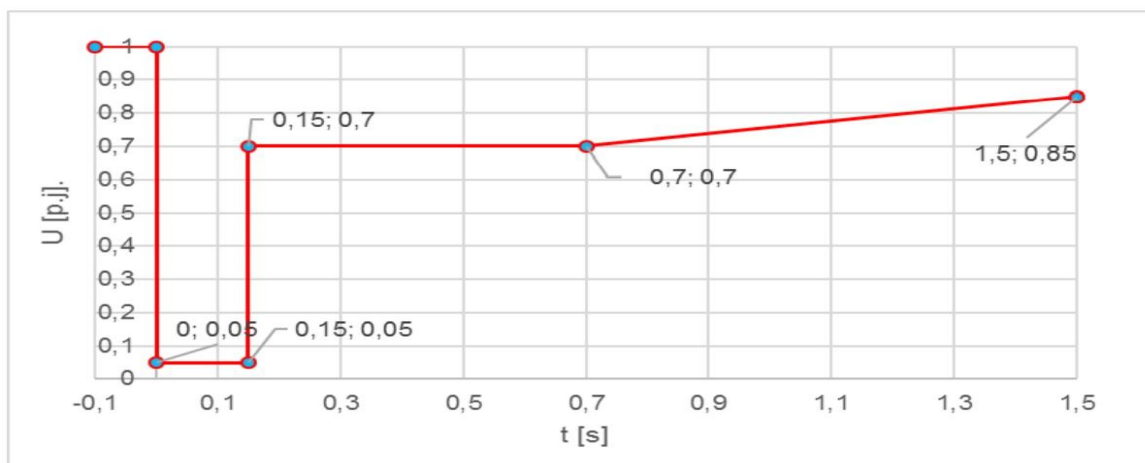
Obrázek č.5 Autonomní charakteristika FRT pro synchronní VM B2, C
